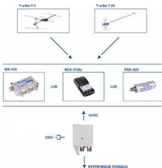
Rys.1. Zastosowanie zasilacza FA-12
